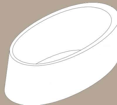
vasca bathtub 170x90x54 cm superficie d'appoggio leaning surface 1,08 mq 350 kg peso weight 310 l capacità capacity
