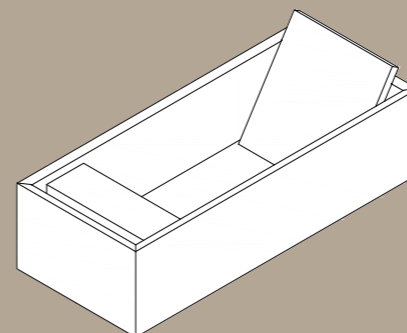
vasca con tracimazione d'acqua interna bathtub with overflowing inside water superficie d'appoggio leaning surface 1,6 mq 400 kg peso weight 400 l capacità capacity
