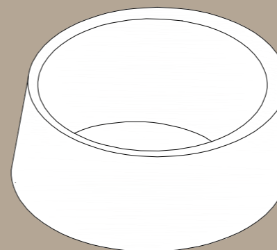
vasca bathtub Ø 140x54 cm superficie d'appoggio leaning surface 1,82 mq 560 kg peso weight 530 l capacità capacity
