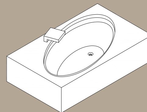
vasca bathtub superficie d'appoggio leaning surface 2,4 mq 440 kg peso weight 220 l capacità capacity
