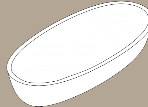
vasca bathtub 200x95x46 cm superficie d'appoggio leaning surface 0,8 mq 350 kg peso weight 280 l capacità capacity
