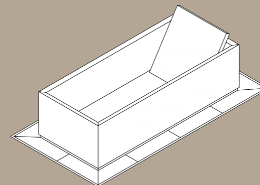
vasca con tracimazione d'acqua esterna bathtub with overflowing outside water superficie d'appoggio leaning surface 1,6 mq 400 kg peso weight 400 l capacità capacity
