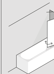
STAR 1 ANTA BATTENTE + LATO FISSO / 1 HINGED DOOR + FIXED SIDE
